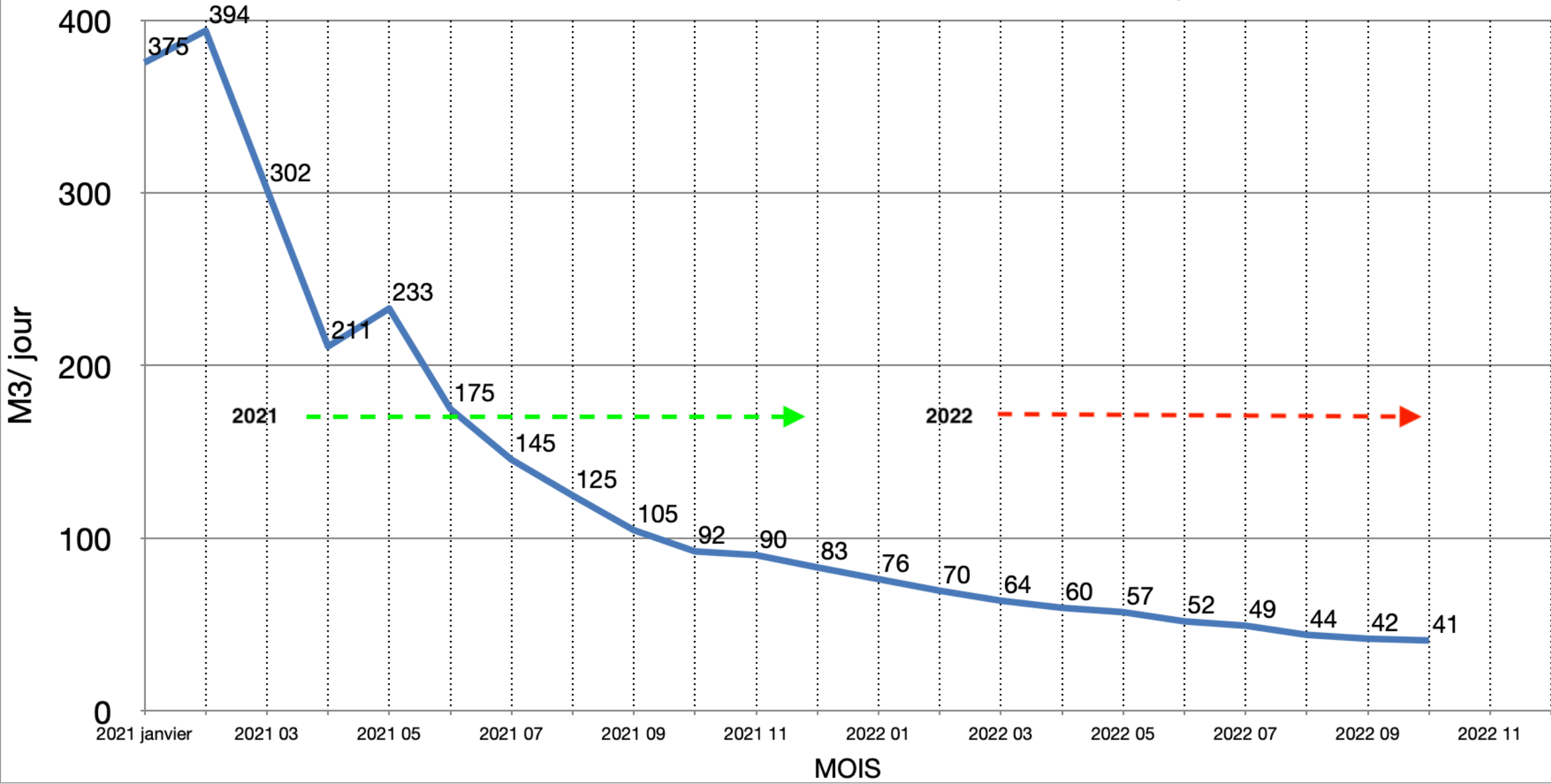
SOURCE du JONCAS. évolution du DEBIT mensuel moyen
